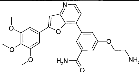
3-(2-Amino-ethoxy)-5-[2-(3,4,5-trimethoxy-phenyl)-furo[3,2-b]pyridin-7-yl]-benzamide
