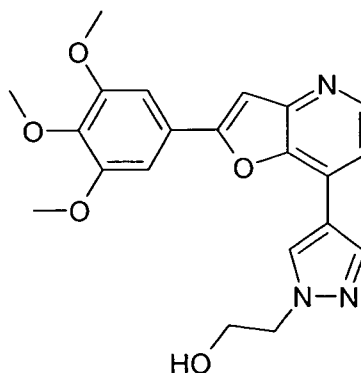
2-{4-[2-(3,4,5-Trimethoxy-phenyl)-furo[3,2-b]pyridin-7-yl]-pyrazol-1-yl}-ethanol
