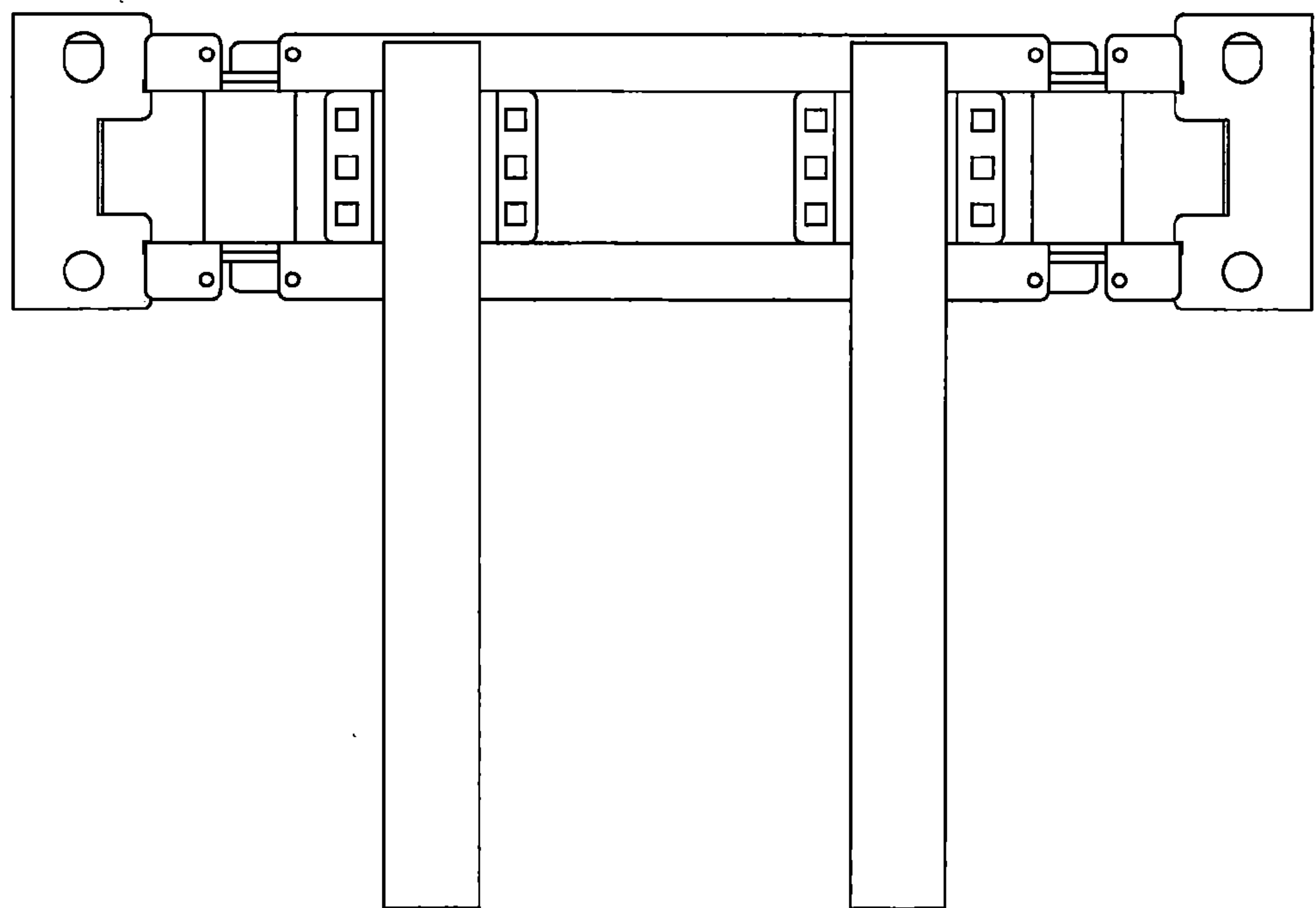
仰視圖
