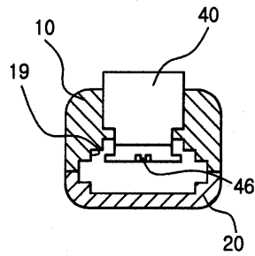
6b B-B'에서 본 단면도
