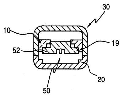
6b B-B'에서 본 단면도
