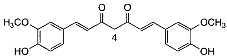
Curcumin
