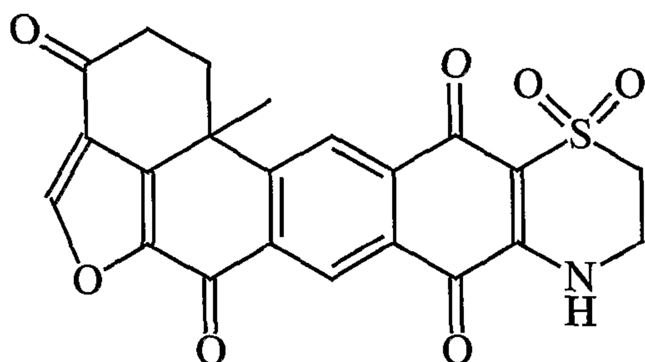
3-Ketoadociaquinone B
