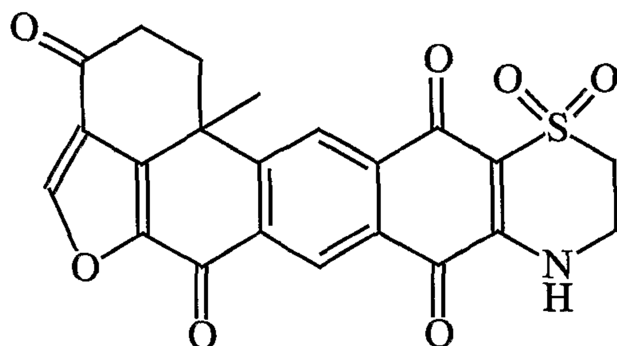
3-Ketoadociaquinone B
