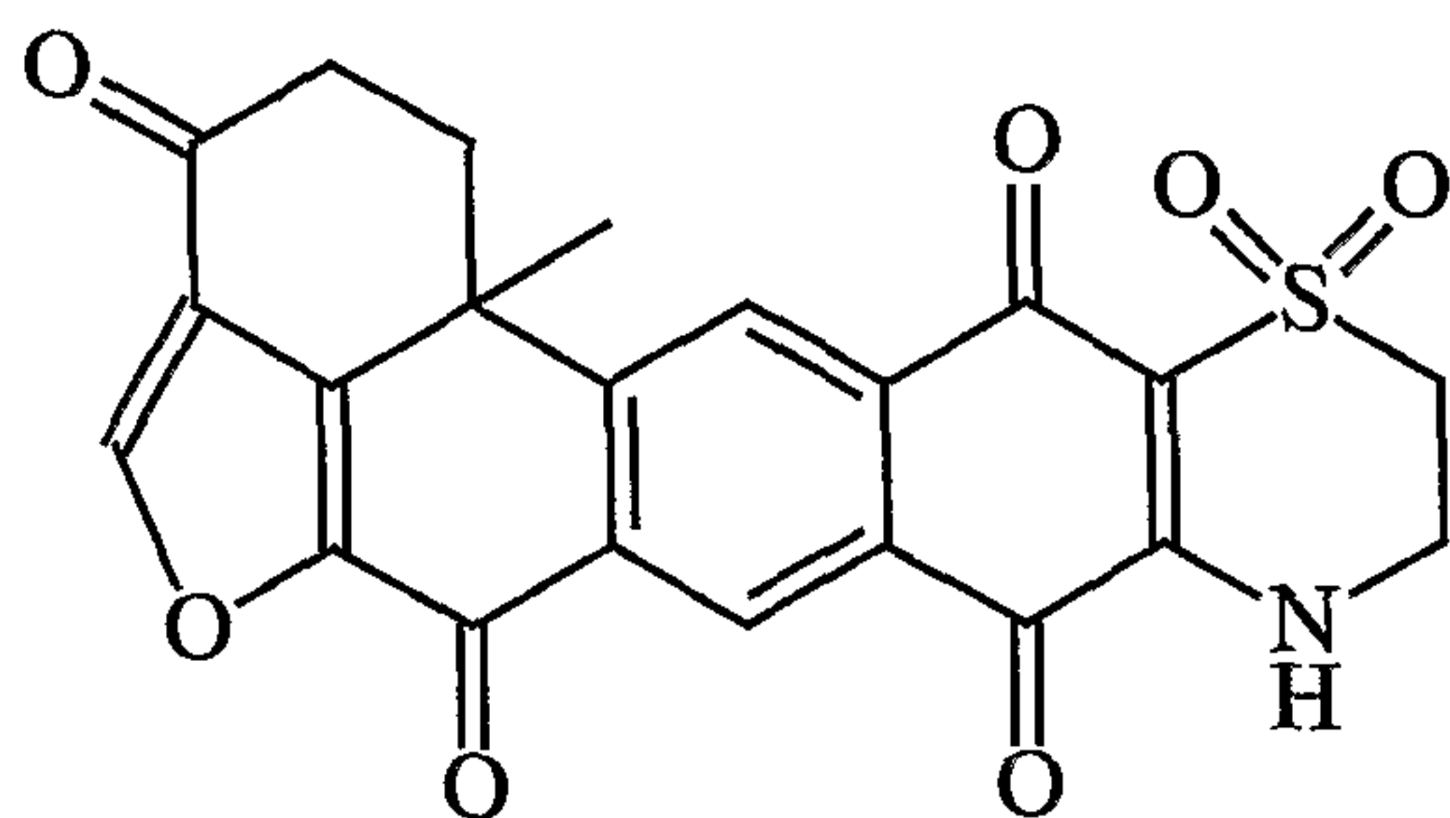
3-Ketoadociaquinone B
