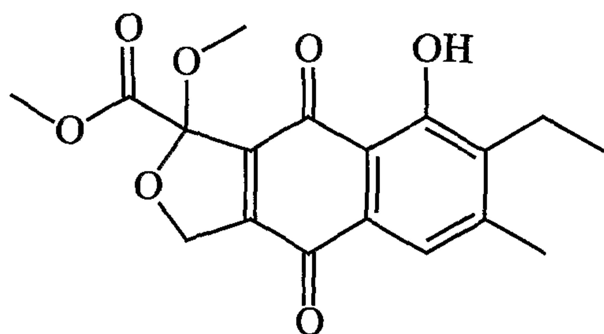
Annulin C
