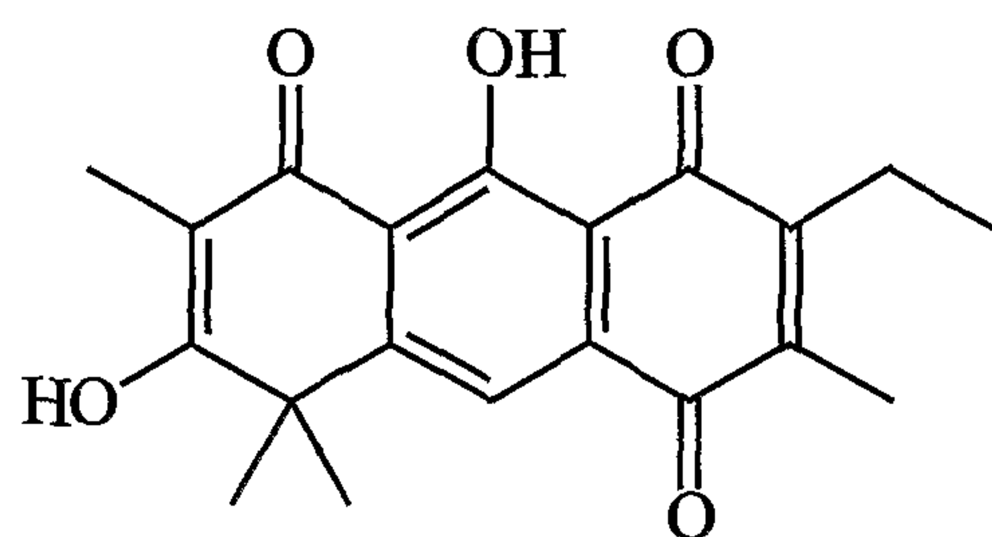
Garveatin E
