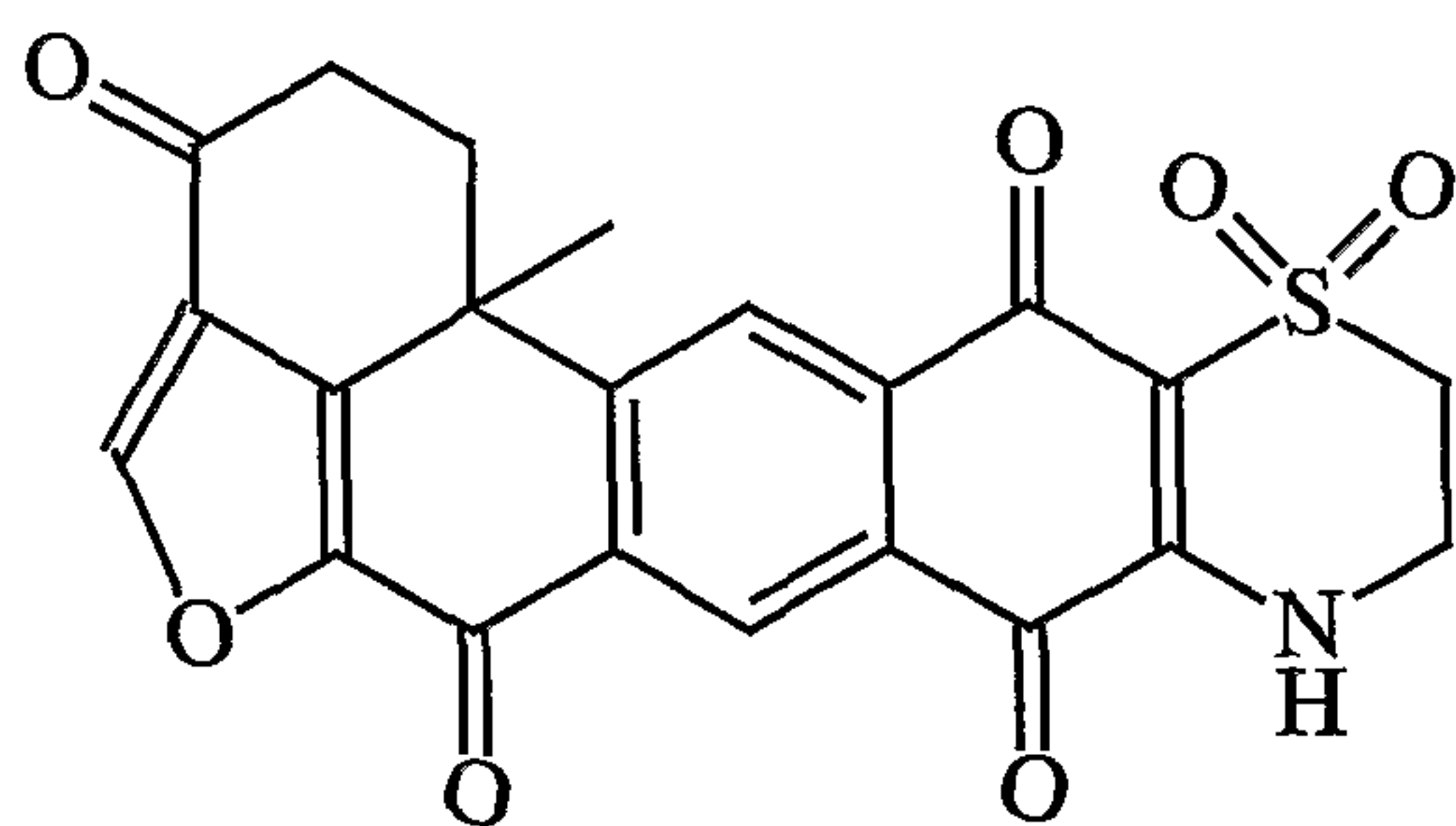
3-Ketoadociaquinone B
