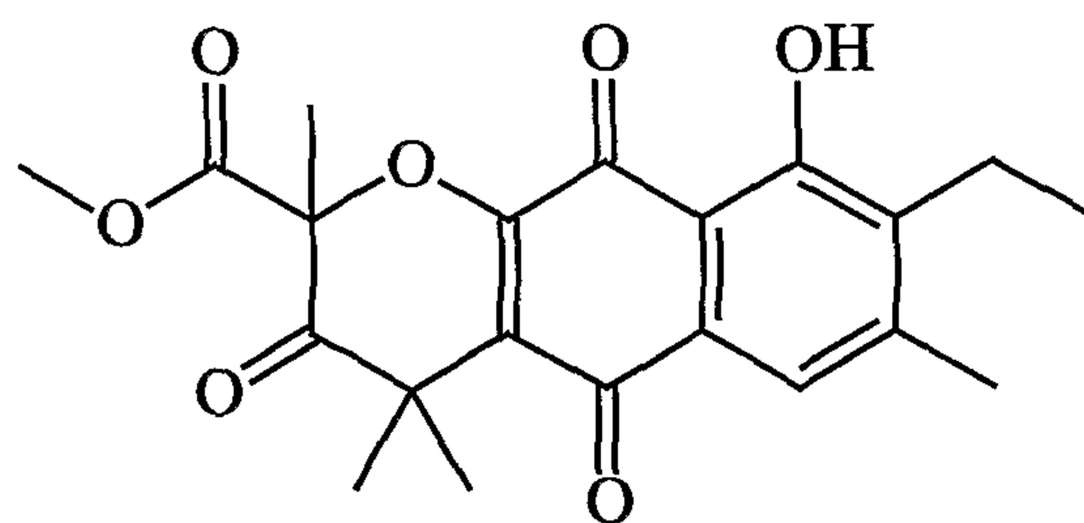
Annulin B
