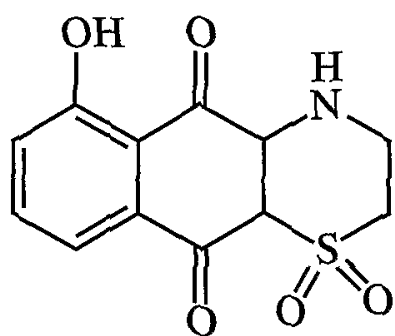
Garveatin E
