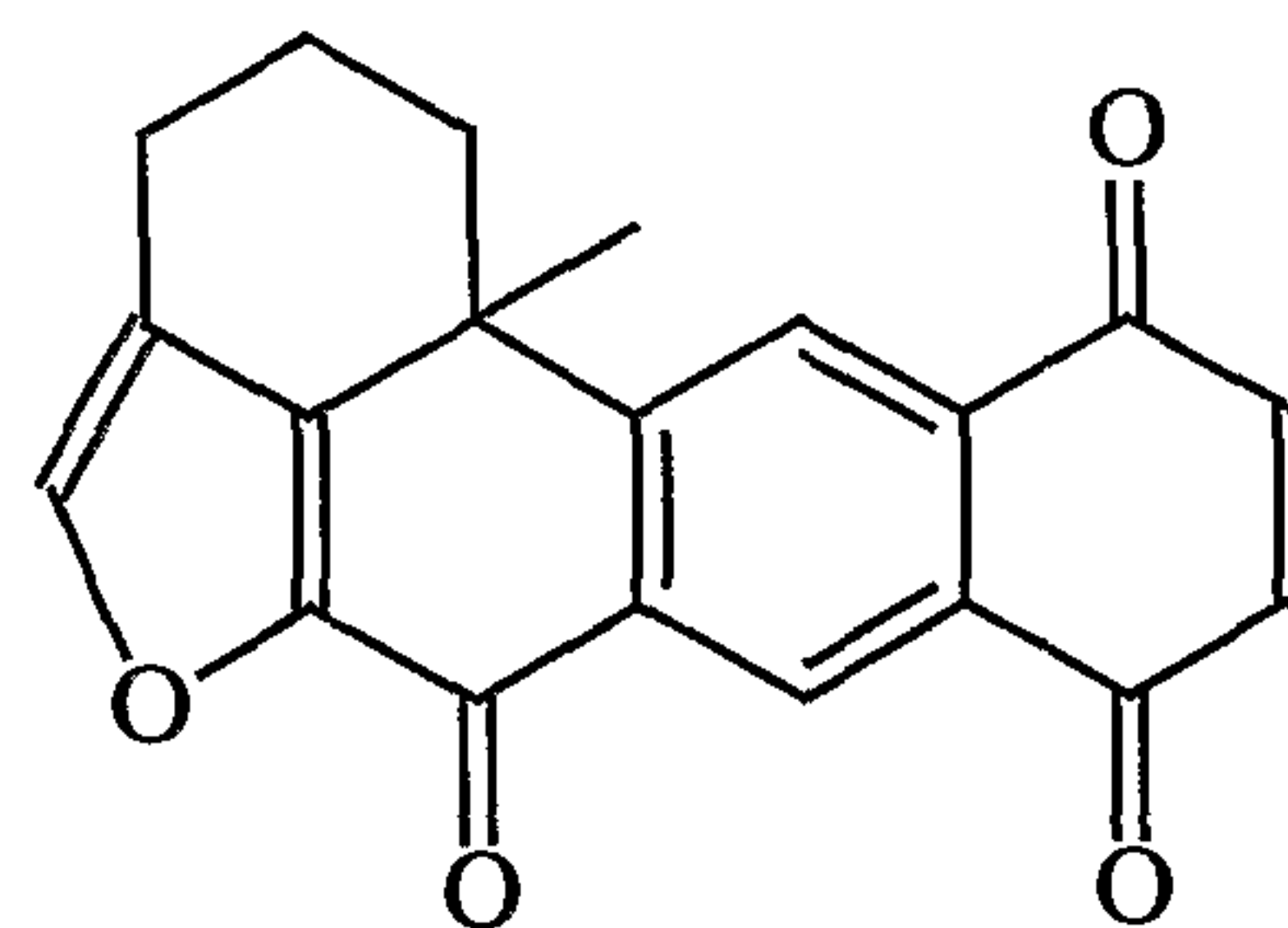
Xestoquinone
