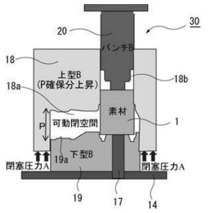
第1アクション 側方押し出し鍛造
