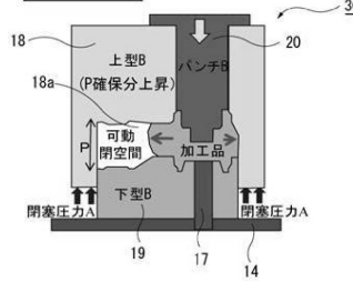
第1アクション 側方押し出し鍛造
