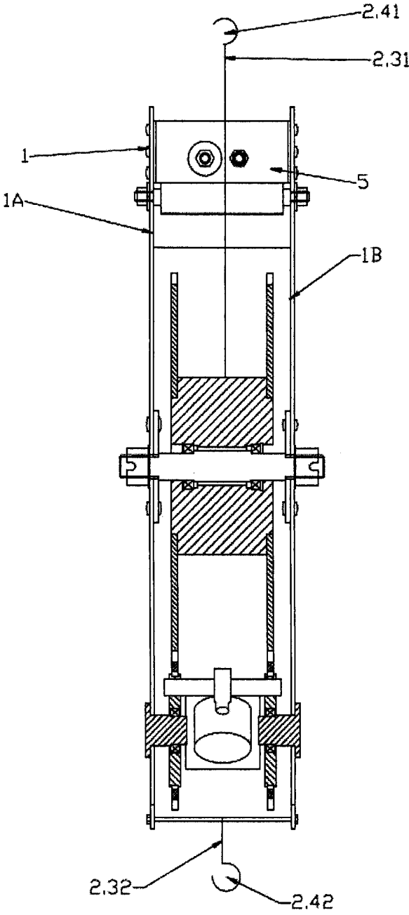
C-C 19 pav.
