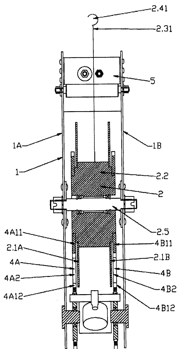
C-C 20 pav.
