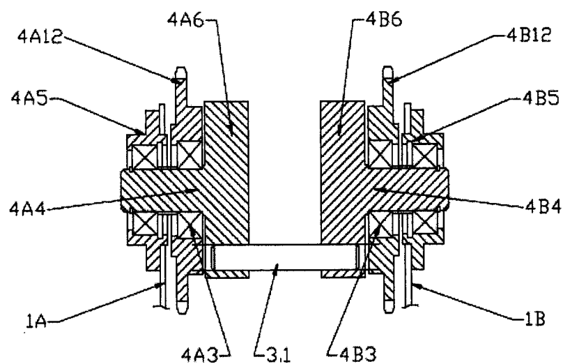
B-B 12 pav.
