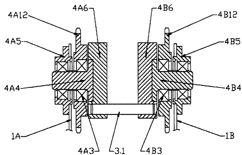
B-B 12 pav.
