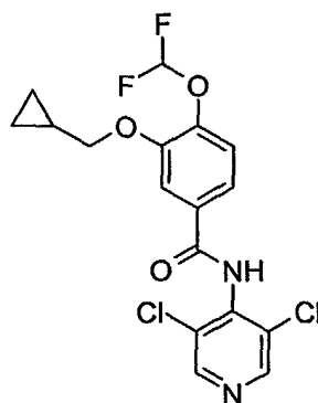
Roflumilast
