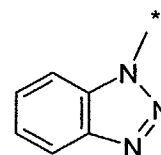
Benzotriazolyl (5.0.16)
