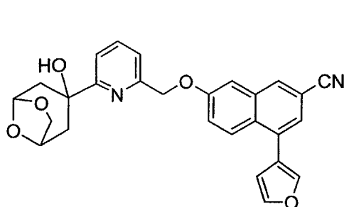
L-739,010
