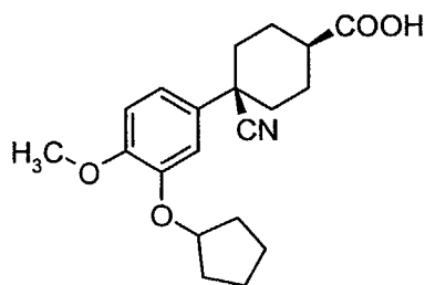
SB-207,499
