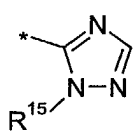
1,2,4-triazol-3-yl
