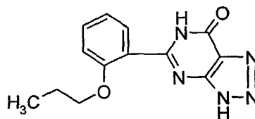
Zaprinast
