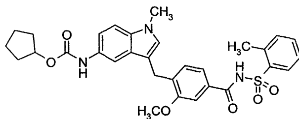
ACCOLATE®
