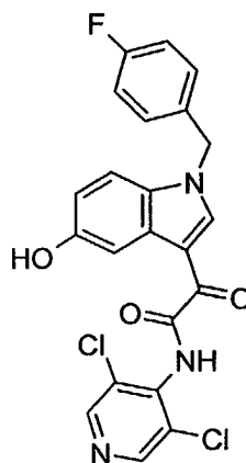
Loteprednol (AWD - 12,281)
