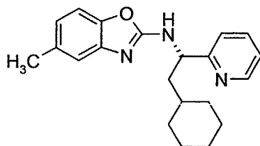
Ontazolast
