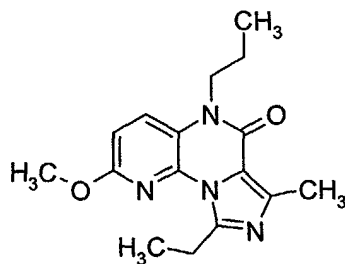
D-22888
