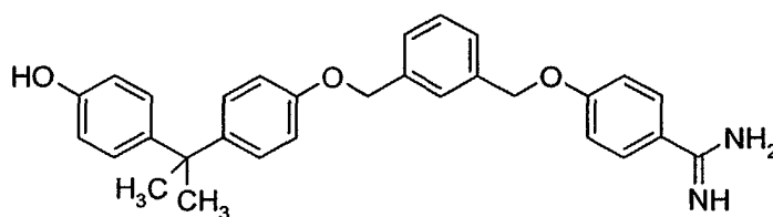
BIIL-260
