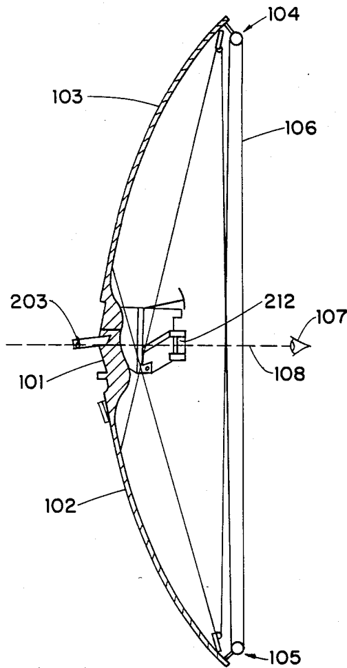
Fig. 1A
