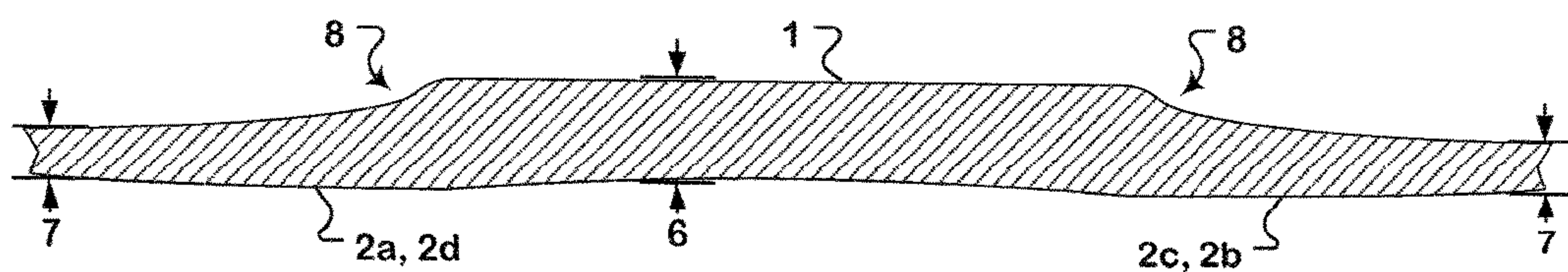
FIG. 9A A-A
