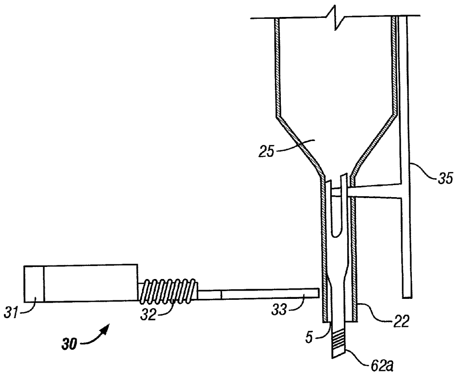
FIG. 13C
