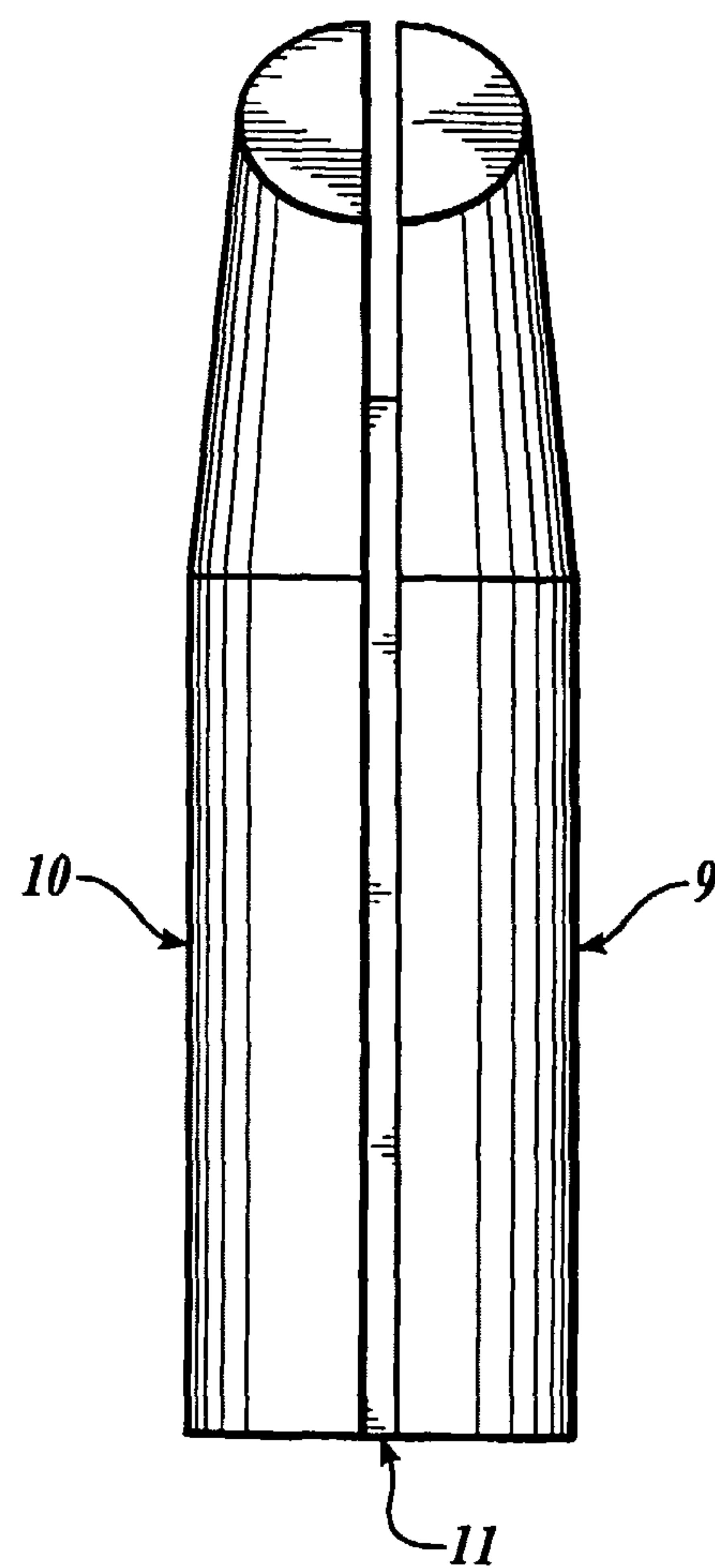
Fig. 2.
