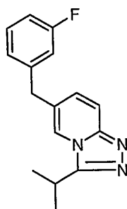
6-(4-fluorobenzyl)-3-isopropyl[1,2,4]triazolo[4,3-a]pyridine
