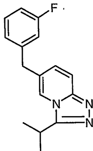
6-(3-fluorobenzyl)-3-isopropyl[1,2,4]triazolo[4,3-a]pyridine
