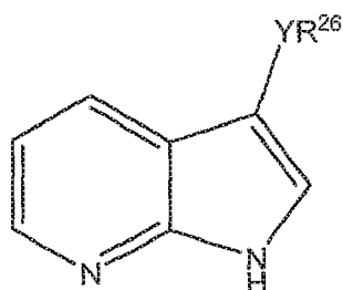
Formula Io
