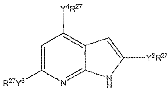
Formula Iu
