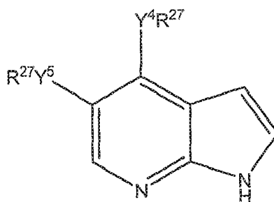
Formula Ij
