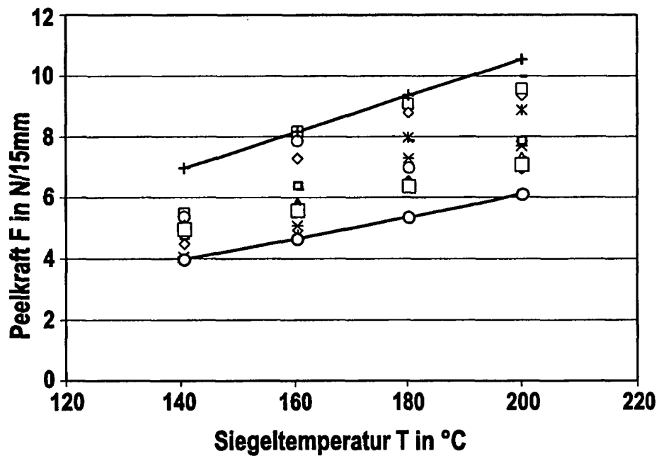
Fig. 5 Zusammenhang zwischen Siegeltemperatur in °C und Peelkraft in N/15mm
