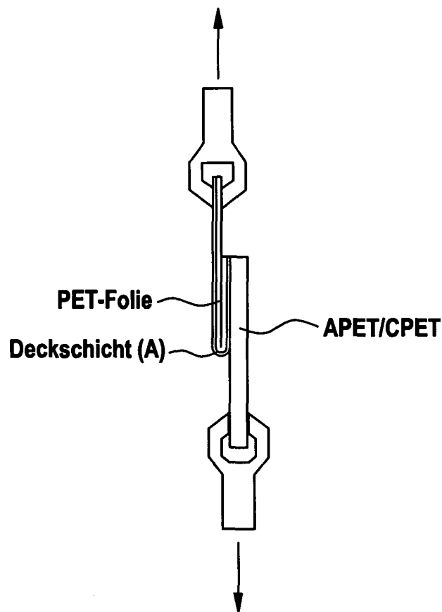
Fig. 2 Anordnung von "peelfähiger" Folie und Streifen einer APET/CPE-Menseschale im Zug-Dehnungs-Messgerät
