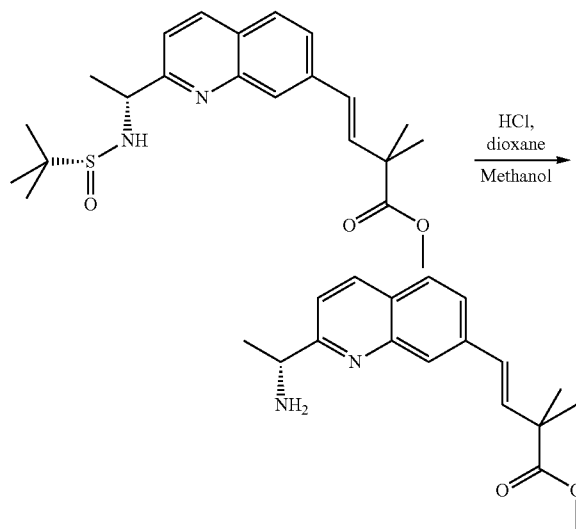
Compound 18e
