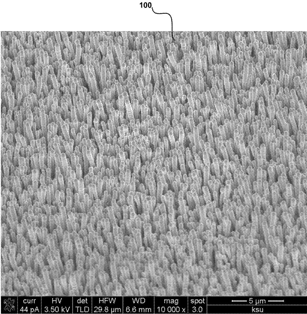
FIG. 11A
