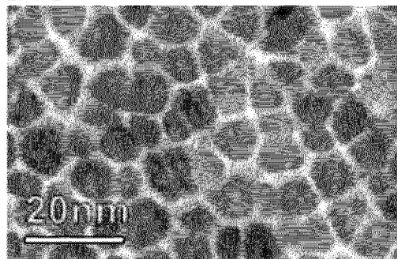
Co-Pt-Cr-TiO 2 -SiO 2
