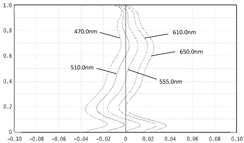
轴向像差
