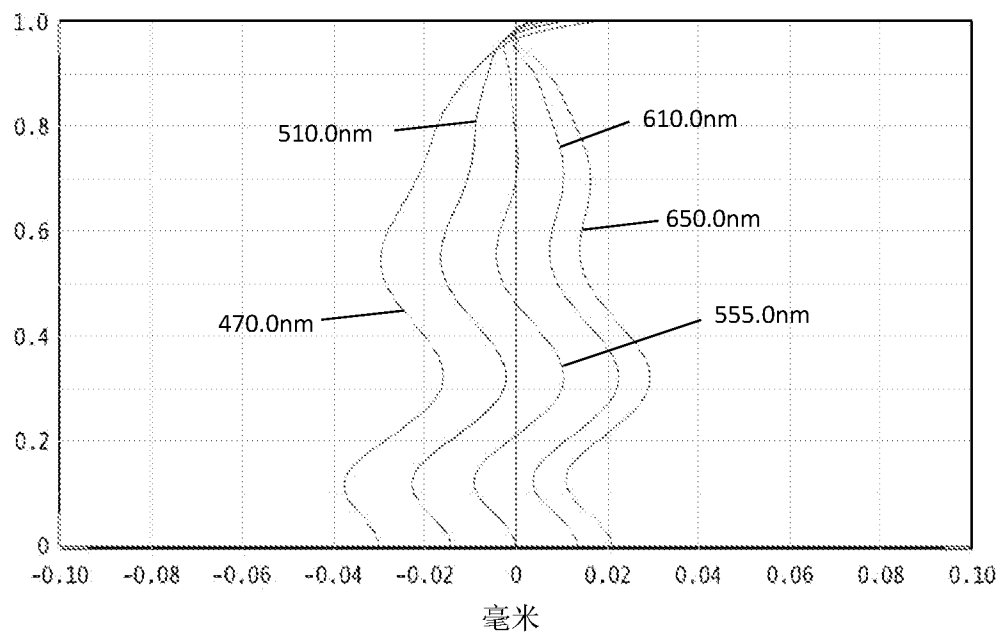
轴向像差
