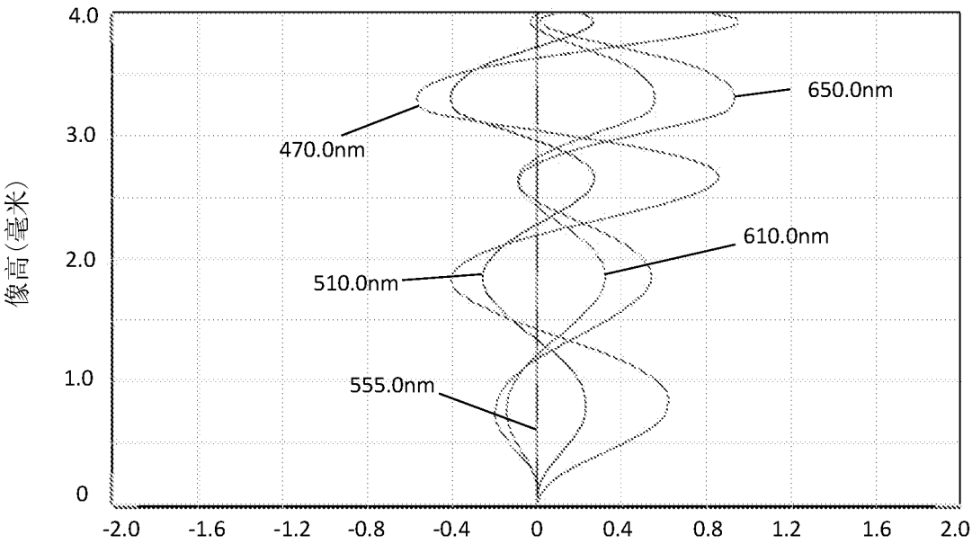
倍率色差
