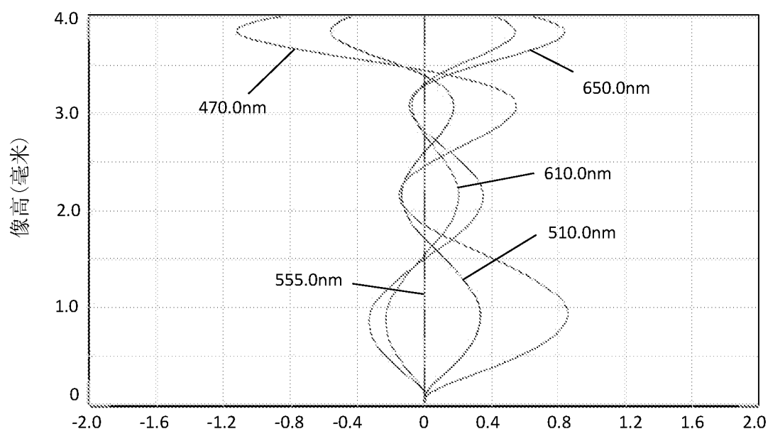
倍率色差
