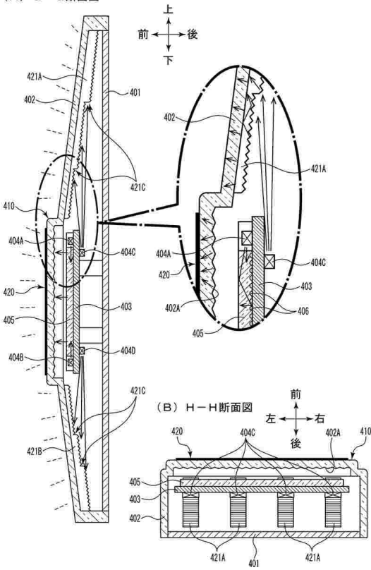
【図16-18】 (A) G-G断面図
