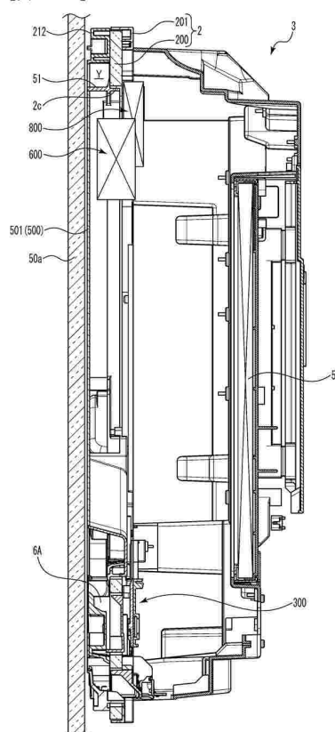
【图16-4】 A—A断面图
