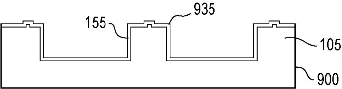
FIG. 9G
