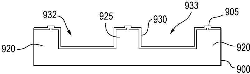
FIG. 9F
