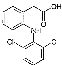
Diclofenac (Ia)
