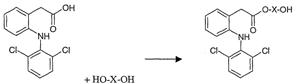
diclofenac (Ia)
