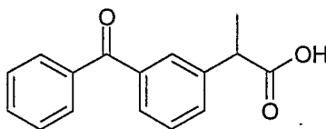
Ketoprofen (Id)
