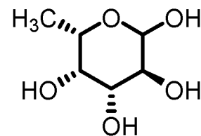
L-fucose;
