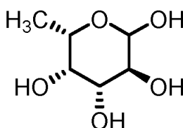
L-fucose
