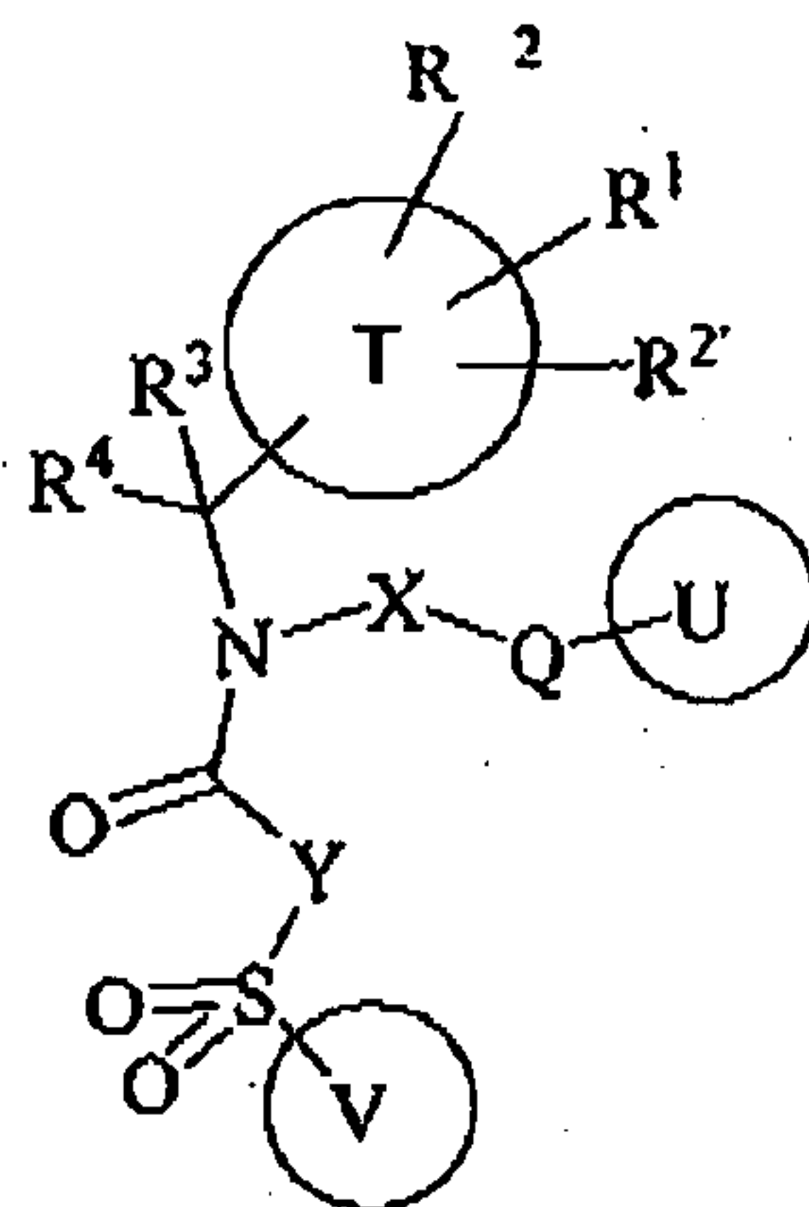
(Ia)
