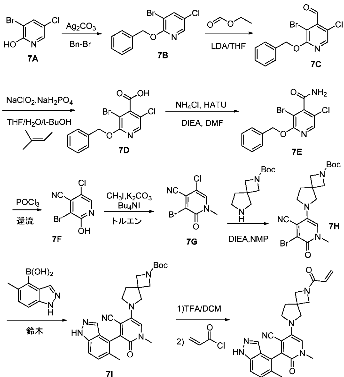
化合物 I-135
