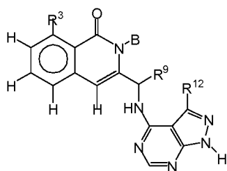
Formula XI-A
