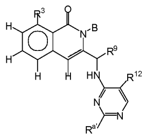
Formula XIV-A
