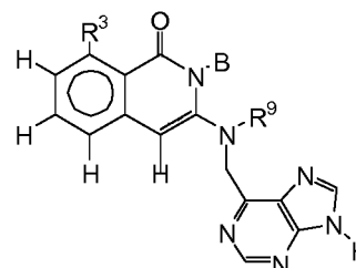
Formula VI-A
