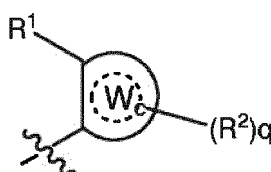
Formule II
