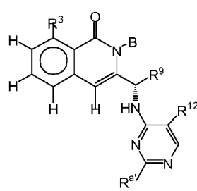
Formula XIV-A2
