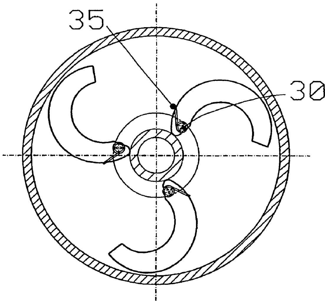
Fig. 4F section A-A
