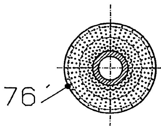
Fig. 7E section F-F
