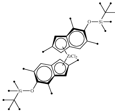
Bis( \eta^5 -2,5,7-trimethyl-6-tert-butyl dimethylsiloxy-1H-indenyl)dichlorozirconium (IV)
