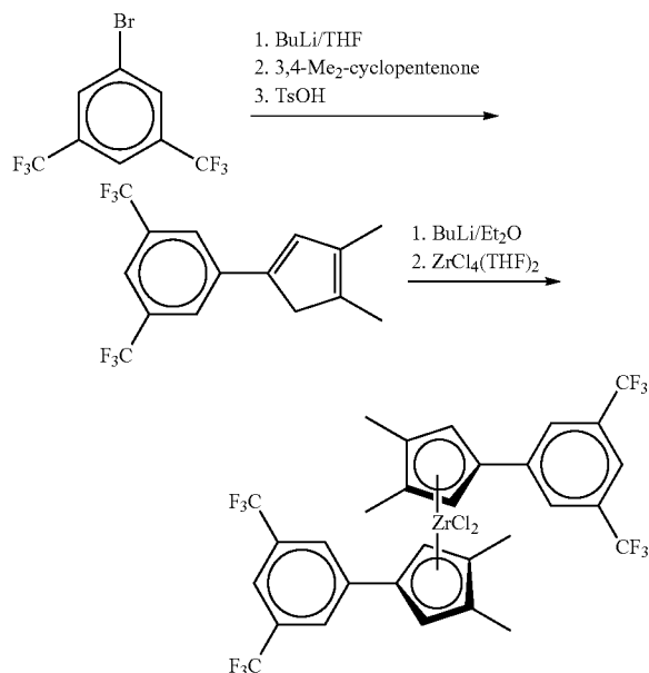
1-(3,4-Dimethyl-1,3-cyclopentadien-1-yl)-3,5-bis(trifluoromethyl)benzene
