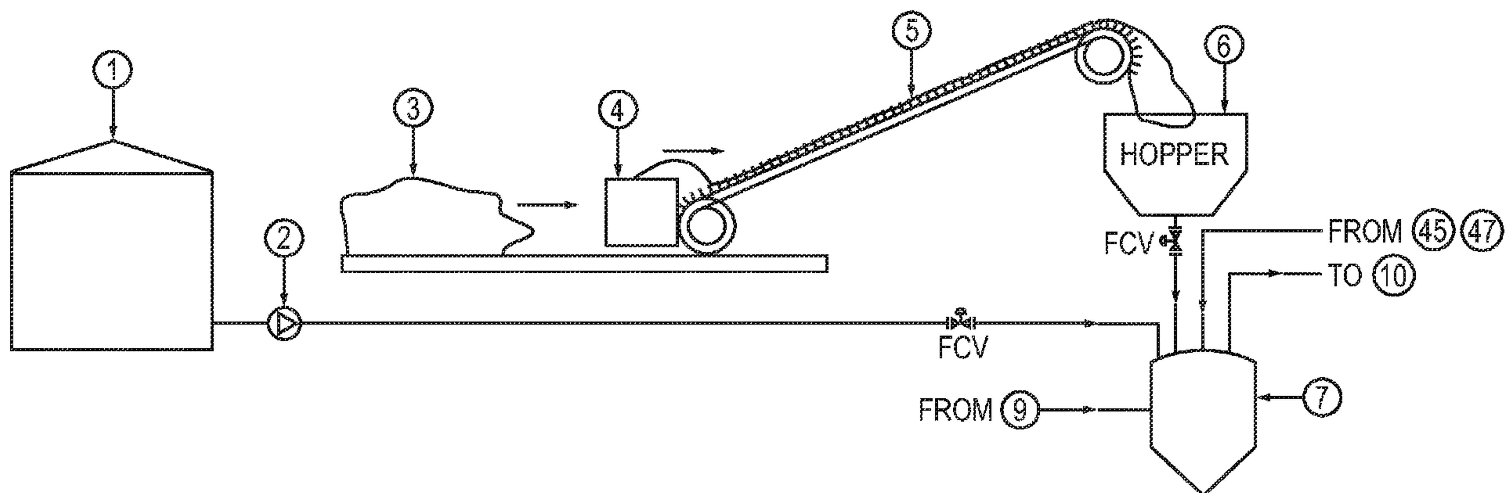
Subsystem-S1
