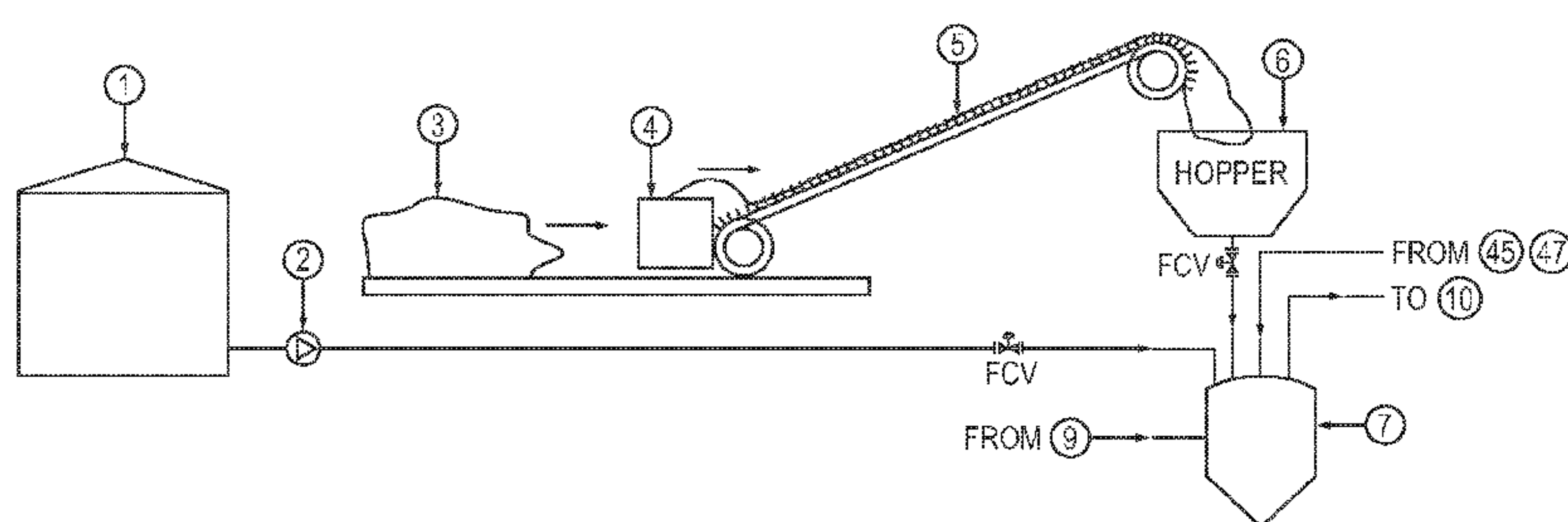
Subsystem-S1
