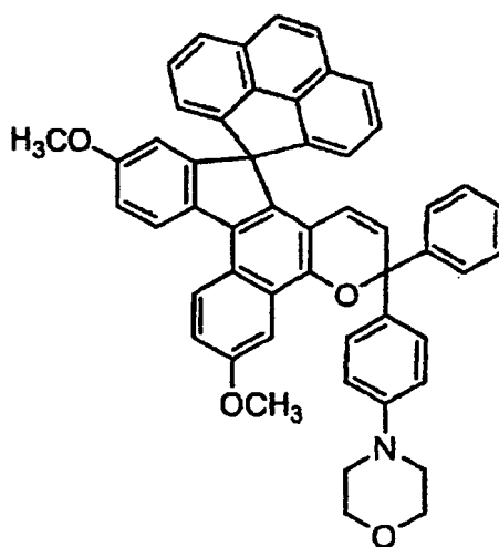
Chromene 1
