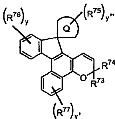
[Chem. 23]
