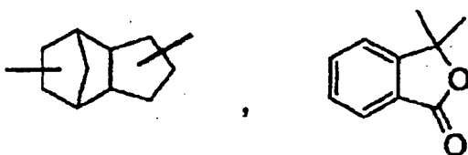
[Chem. 6]
