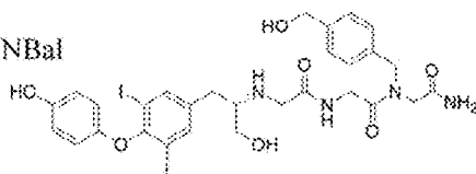
T2AA-NEal-NTyr
