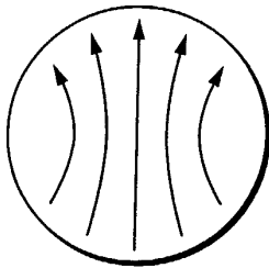
TE11 MODE
