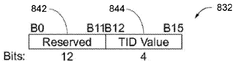
Per TID Info Field
