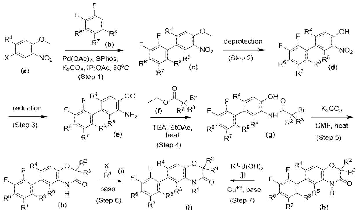
Scheme 1a
