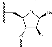
2'-F-ANA (arabino)
