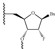
2'-F (ribo)
