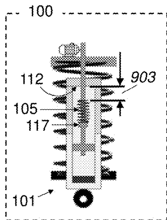
Design FIG. 12A
