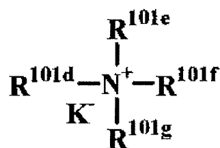
(P1a-3)
