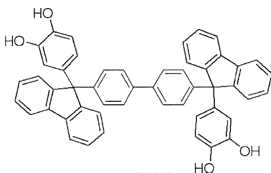
(X-11)
