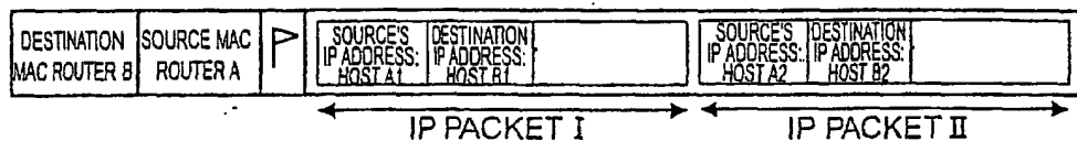
ETHERNET FRAME VI
