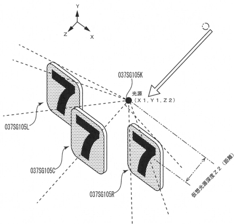
原理図 4 (A)
