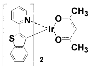
Btp 2 Ir(acac)
