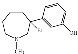
Meptazinol
