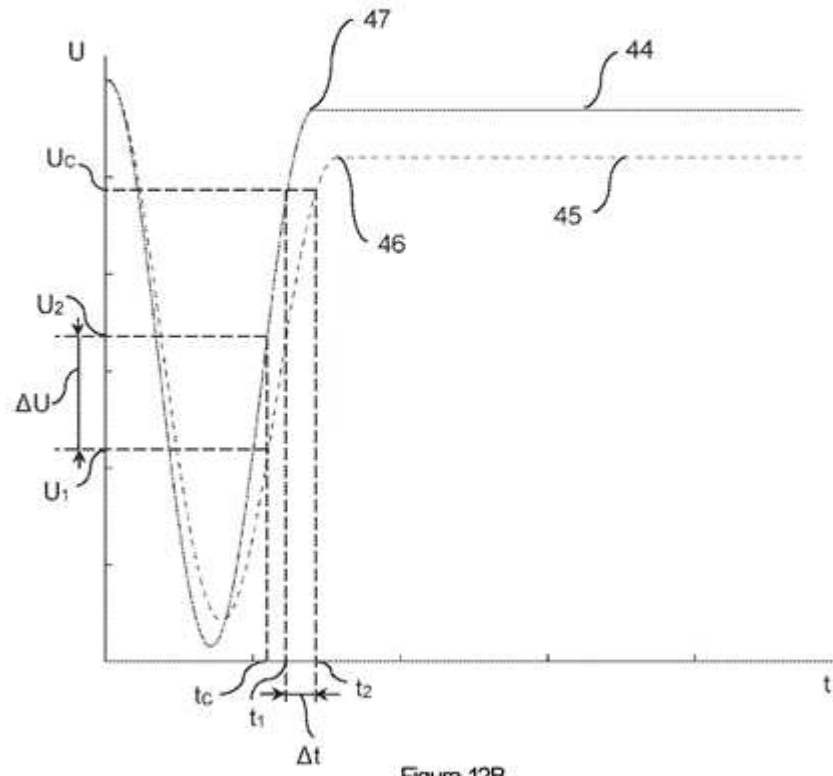
Figura 12B
