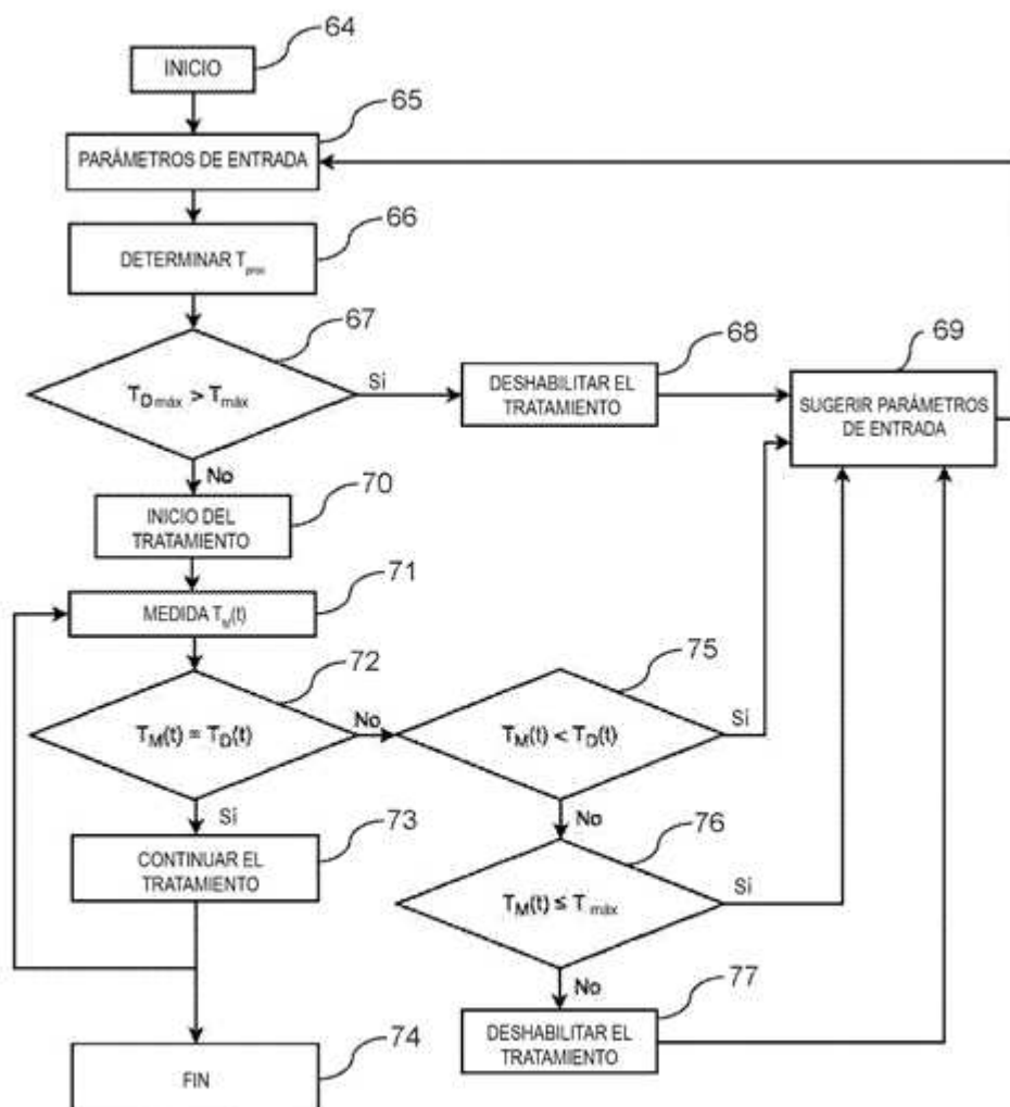
Figura 15
