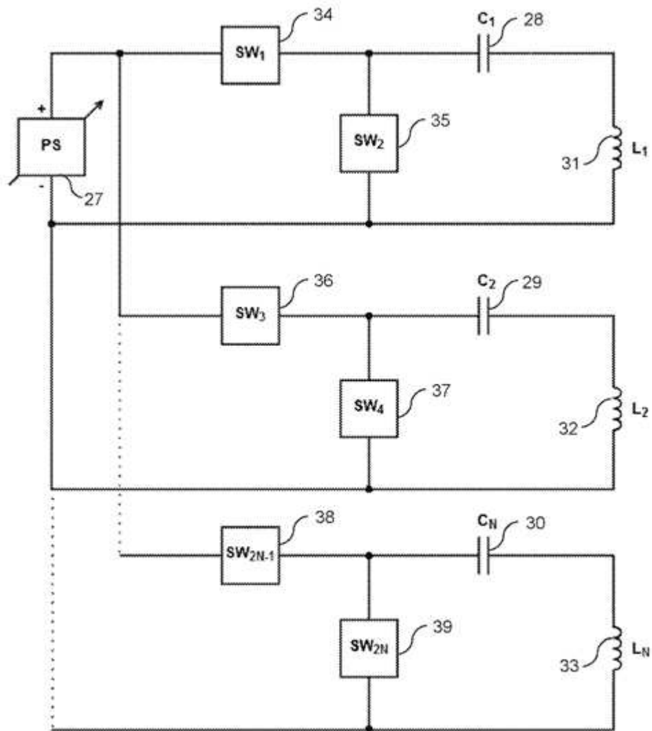
Figura 9
