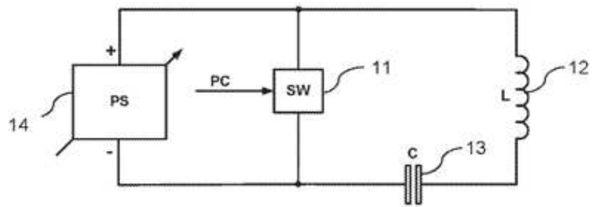
Figura 4B
