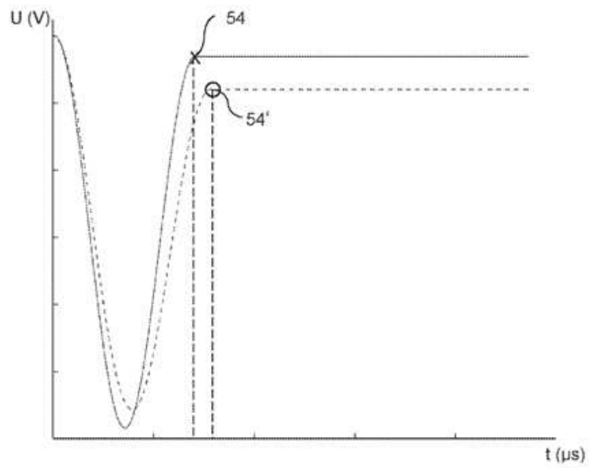
Figura 12E
