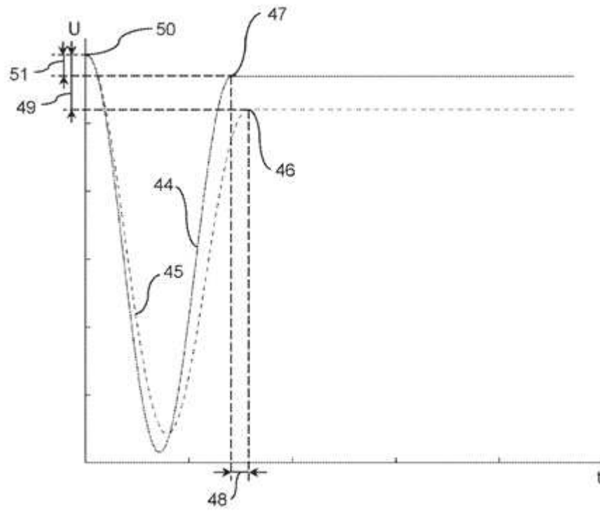
Figura 12A
