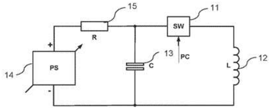
Figura 4A
