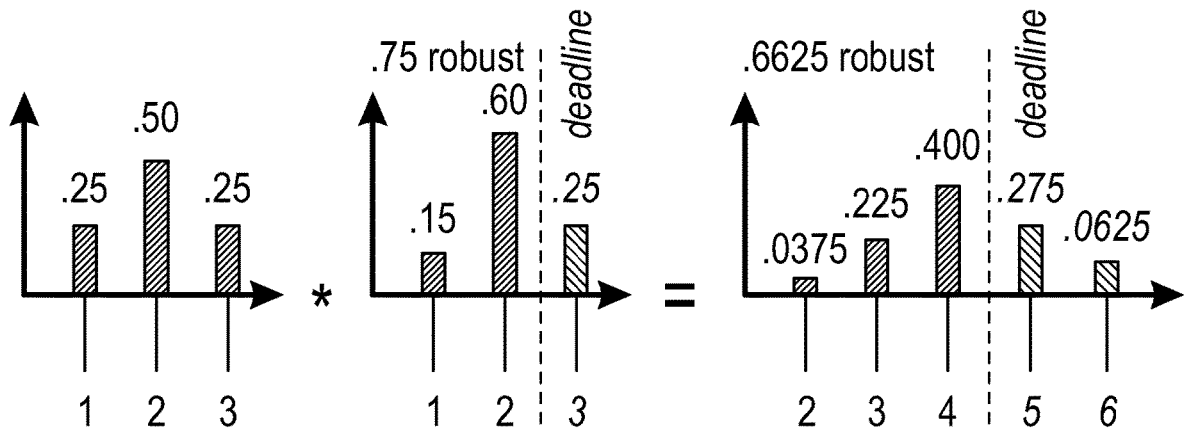
(b) Left Skew
