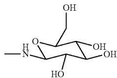
(2-Aminoglucose residue)
