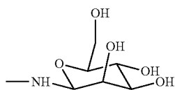
(2-Aminomannose residue)
