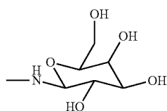
(2-Aminogalactose residue)
