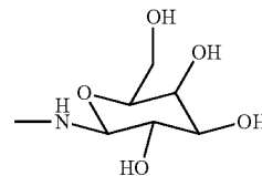
(2-Aminogalactose residue)
