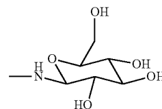
(2-Aminoglucose residue)
