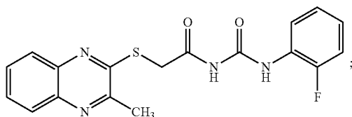
N-((3-fluorophenyl)carbamoyl)-2-((3-methylquinoxalin-2-yl)thio)acetamide (3v)
