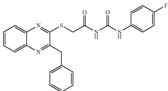
2-((3-benzylquinoxalin-2-yl)thio)-N-((4-fluorophenyl)carbamoyl)acetamide (3ad)
