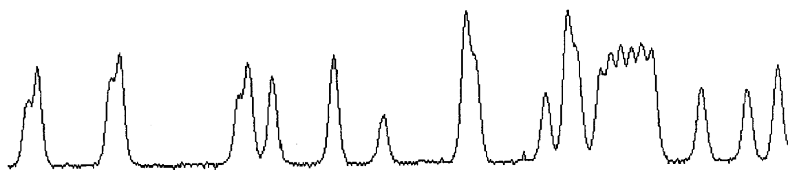
DTAMRA-2-labeled ddCTP using a propargyl-1-ethoxyamido linker
