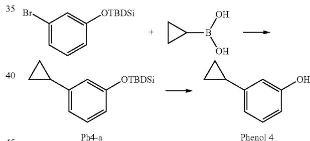
Step a) Tert-butyl(3-cyclopropylphenoxy)dimethylsilane (Ph4-a)
