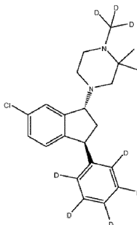
(1 R , 3 S ) - (IV)
