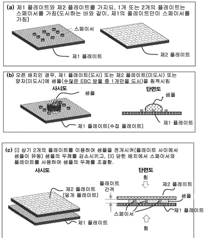
SiEBC(싱글 드롭 EBC 수집기/분석기) 실시형태의 도면
