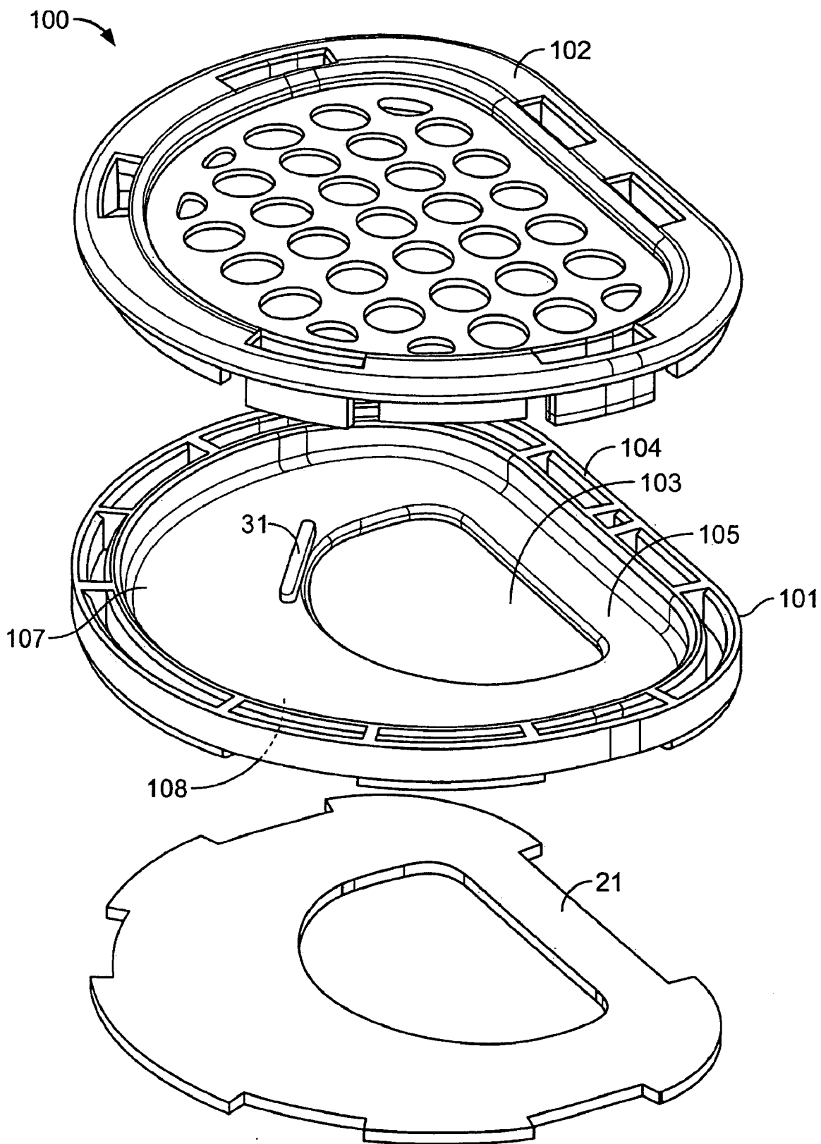
FIG. 10B
